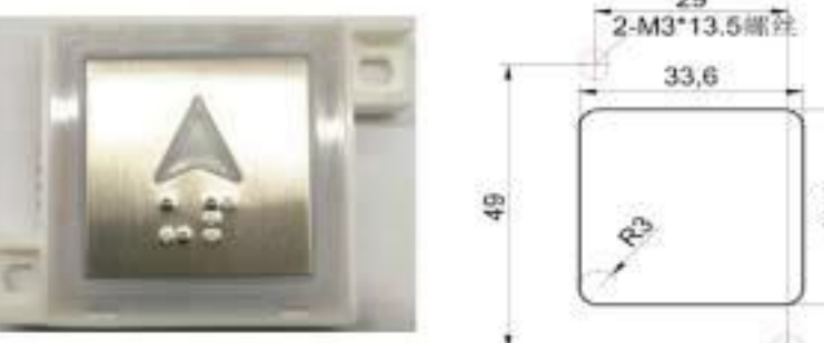
SH-EPB013-F
